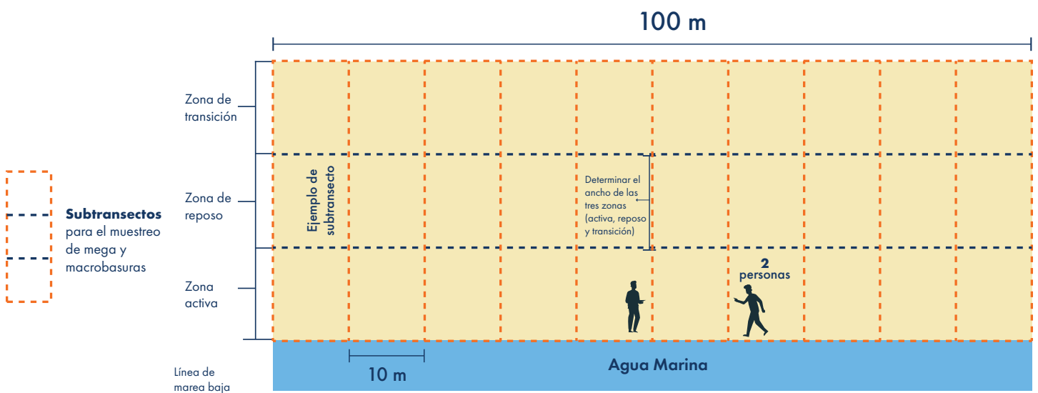
Figura 17. Esquema del método sistemático de basuras marinas en playas arenosas colombianas.
